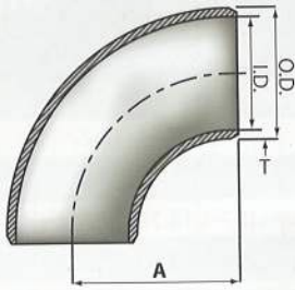
90° elbow long radius
